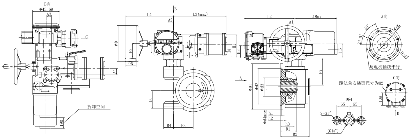
SMC-00~2Ex (IN) 带HBC外形及连接尺寸
